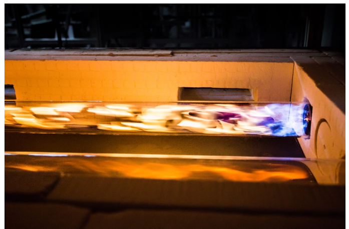
Bild 2: Verbrennung in einem Strahlheizrohr
