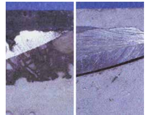
ALUGARD CE-Probe mit ARA (rechts) und ohne ARA (links)
