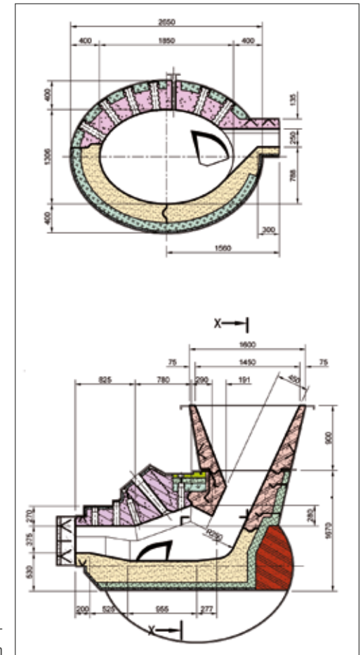
Ofen- zeichnungen
