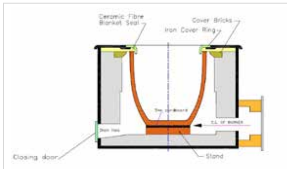
Statischer Ofen
